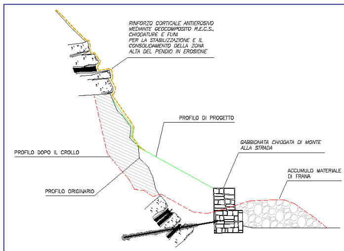
▲ Sezione schematica di intervento
