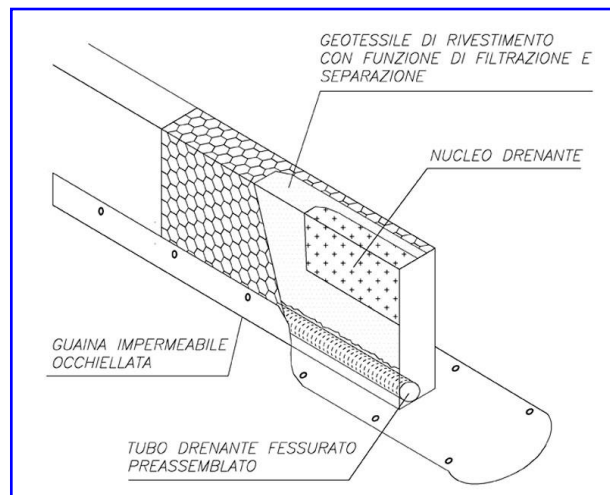
Figura 1 - Pannello drenante prefabbricato Gabbiodren®T - schema
